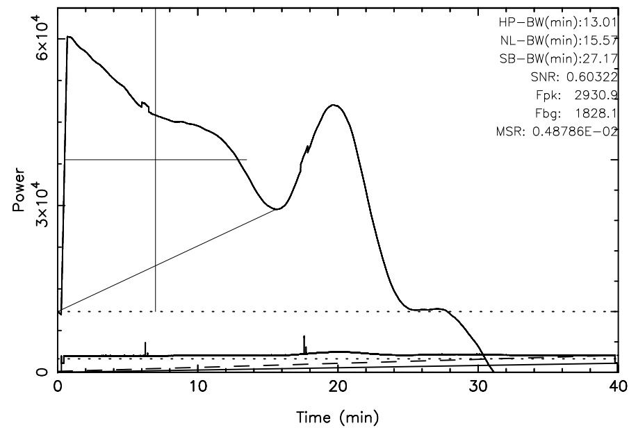
TOYOKAWA 3C348 2023/07/07(188)21:21:55-22:01:55JST
