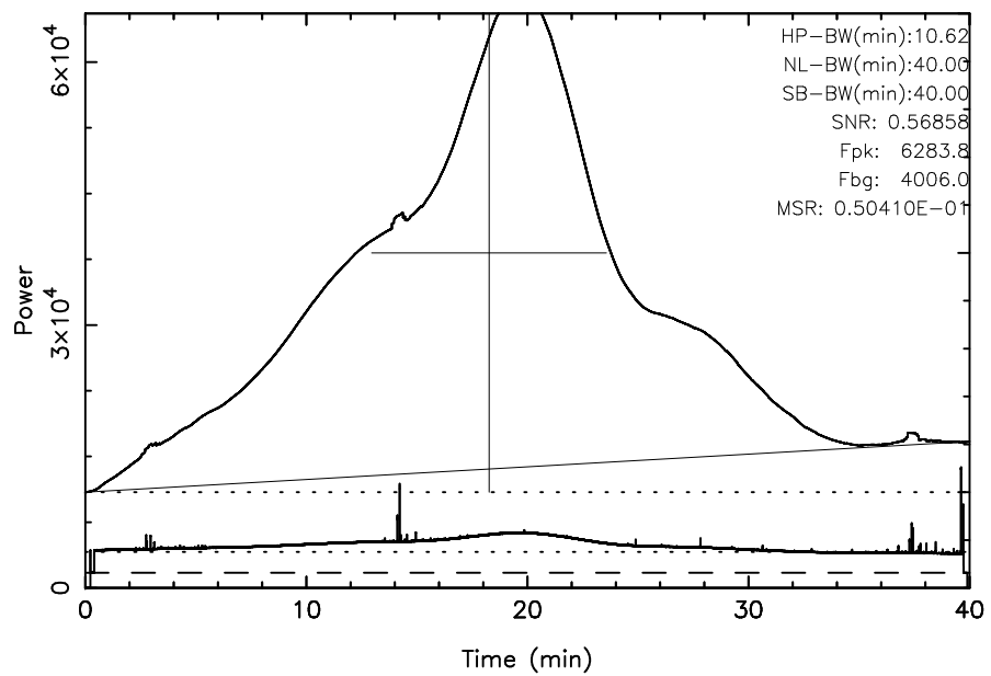
TOYOKAWA 3C392 2023/07/19(200)22:39:23-23:19:23JST
