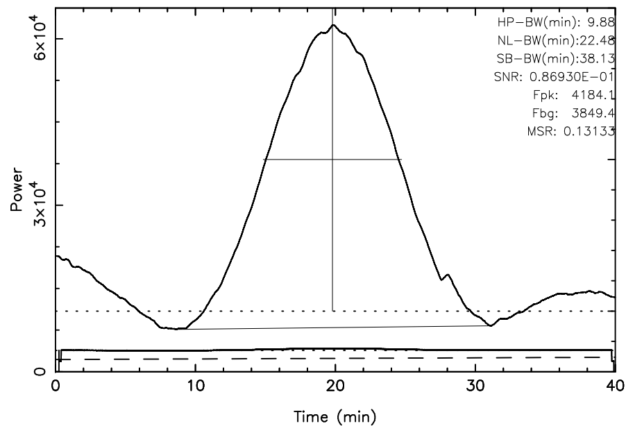
TOYOKAWA 3C10 2023/07/27(208)03:40:24-04:20:24JST
