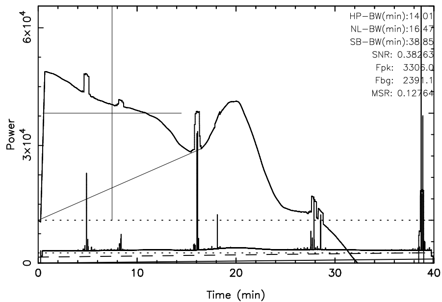
TOYOKAWA 3C348 2023/07/27(208)20:03:17-20:43:17JST
