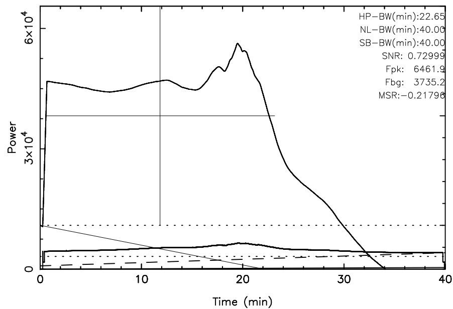
TOYOKAWA 3C392 2023/07/27(208)22:07:55-22:47:55JST
