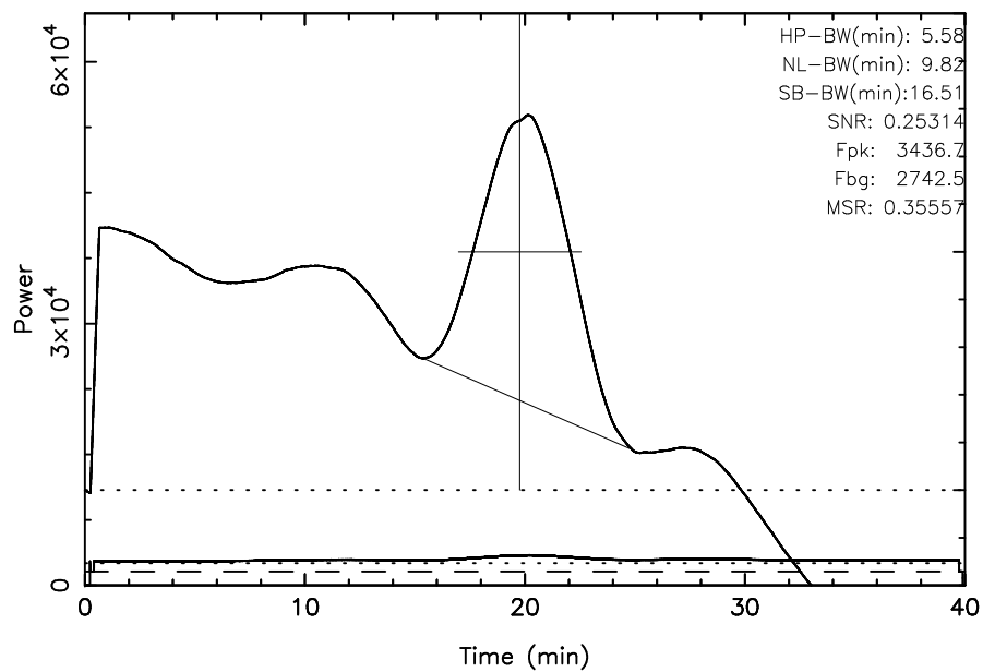
TOYOKAWA 3C348 2023/08/02(214)19:39:41-20:19:41JST
