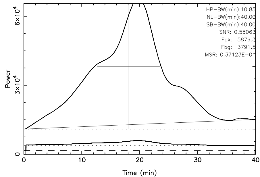
TOYOKAWA 3C392 2023/08/02(214)21:44:20-22:24:20JST
