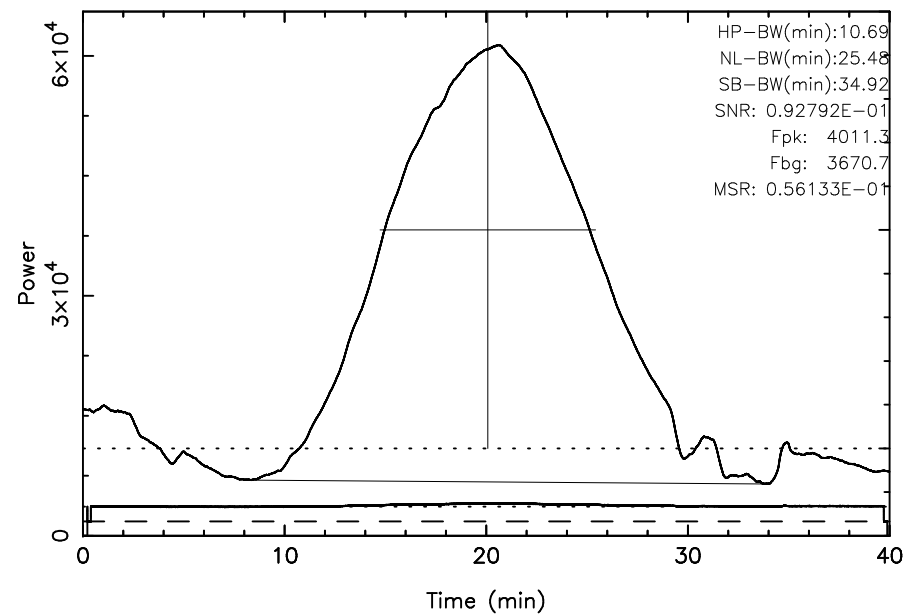
TOYOKAWA 3C10 2023/08/02(214)03:16:49-03:56:49JST
