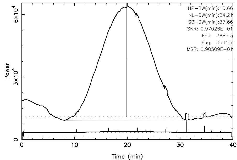
TOYOKAWA 3C10 2023/08/14(226)02:29:38-03:09:38JST
