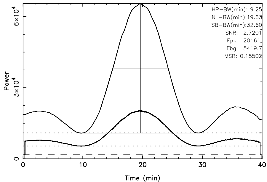
TOYOKAWA 3C461 2023/08/14(226)01:27:30-02:07:30JST
