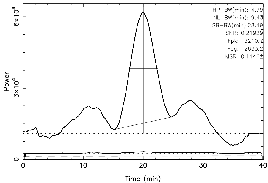
TOYOKAWA 3C348 2023/08/14(226)18:52:30-19:32:30JST
