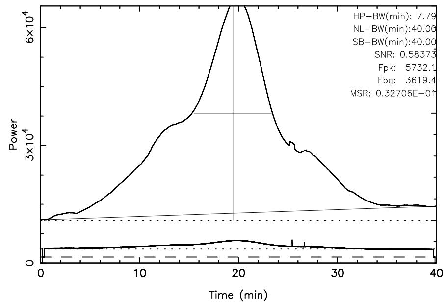
TOYOKAWA 3C392 2023/08/14(226)20:57:09-21:37:09JST
