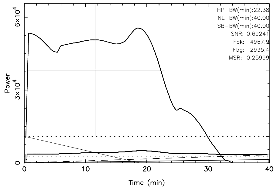
TOYOKAWA 3C392 2023/08/18(230)20:41:25-21:21:25JST
