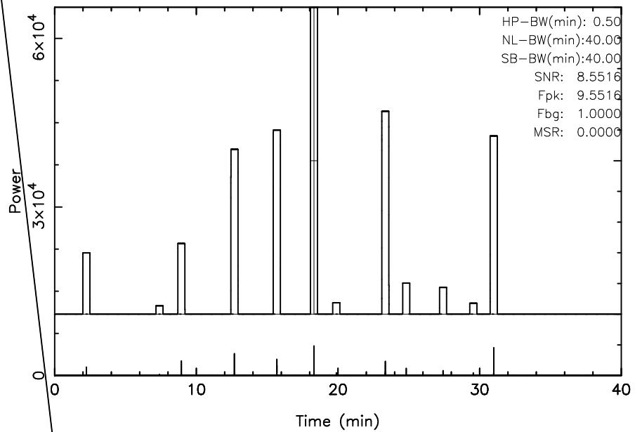
TOYOKAWA 3C348 2023/08/26(238)18:05:20-18:45:20JST
