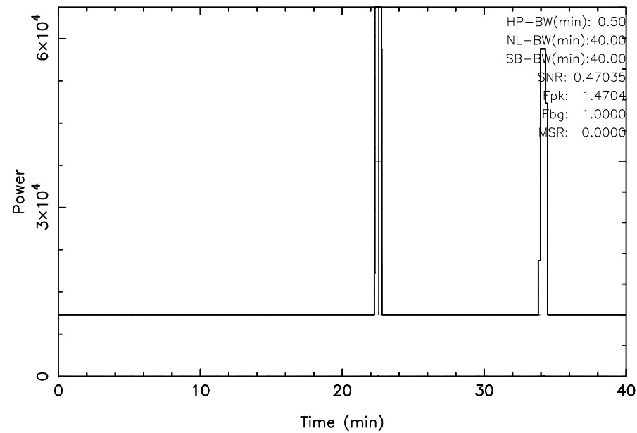
TOYOKAWA 3C10 2023/08/26(238)01:42:27-02:22:27JST
