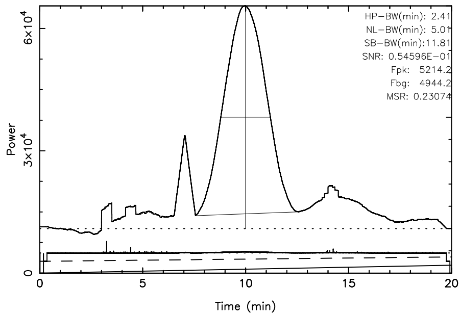
FUJI 3C123 2023/09/07(250)05:16:25-05:36:25JST
