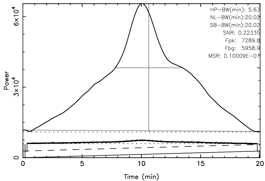
FUJI 3C392 2023/09/07(250)19:32:46-19:52:47JST
