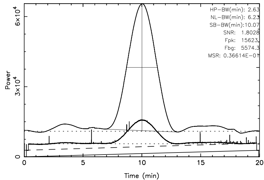
FUJI 3C405 2023/09/07(250)20:35:37-20:55:37JST
