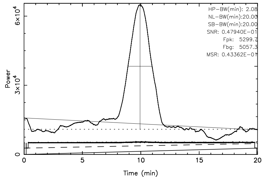
FUJI 3C353 2023/09/07(250)17:57:29-18:17:29JST
