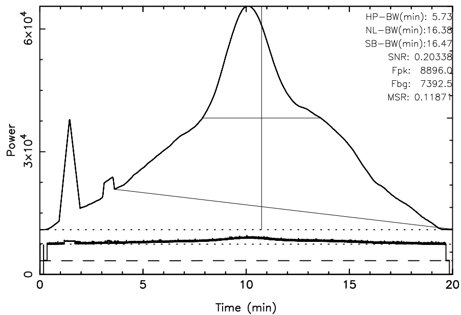
FUJI 3C392 2023/09/25(268)18:22:01-18:42:01JST
