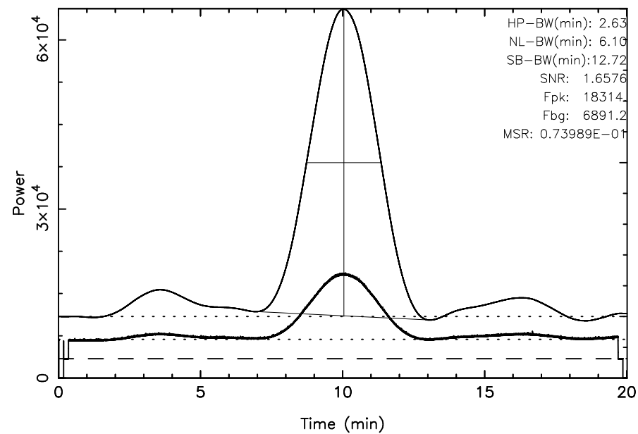
FUJI 3C405 2023/09/25(268)19:24:49-19:44:50JST
