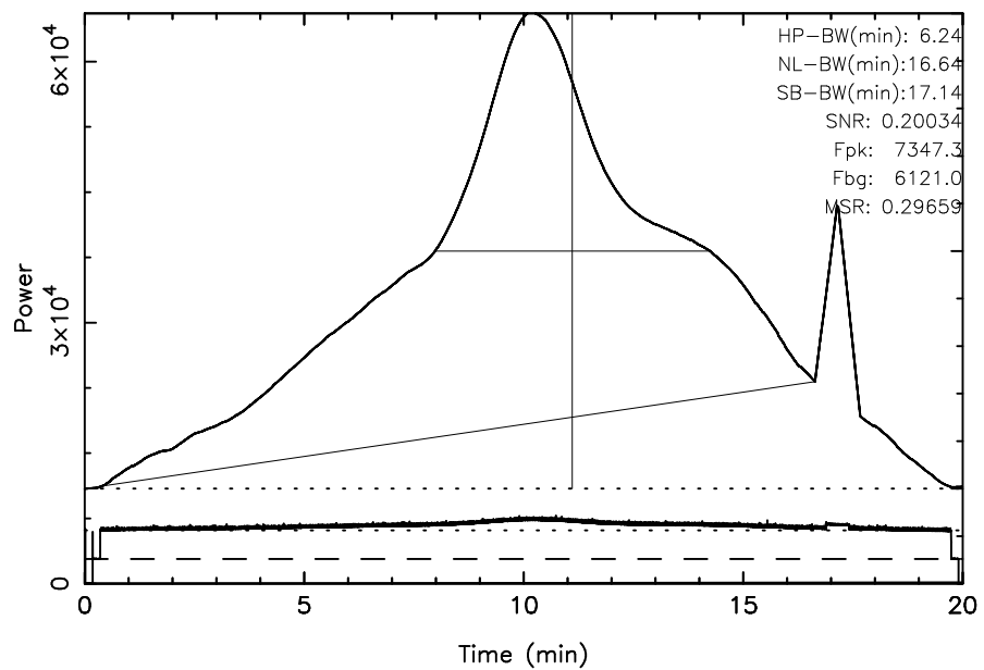
FUJI 3C392 2023/09/29(272)18:06:18-18:26:18JST
