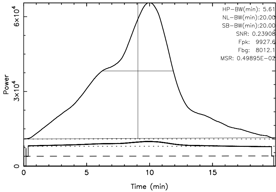
KISO 3C392 2023/09/29(272)18:06:18-18:26:18JST
