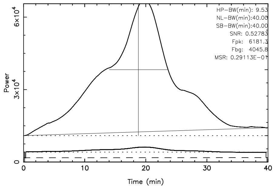
TOYOKAWA 3C392 2023/09/02(245)19:42:27-20:22:27JST
