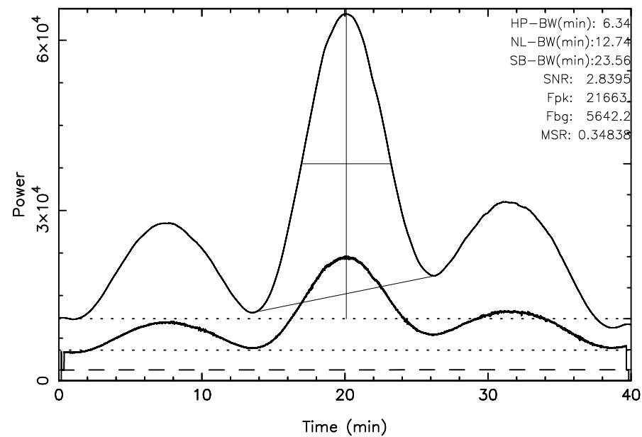
TOYOKAWA 3C405 2023/09/02(245)20:45:16-21:25:16JST
