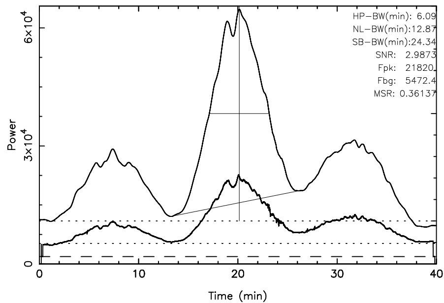
TOYOKAWA 3C405 2023/09/03(246)20:41:20-21:21:20JST
