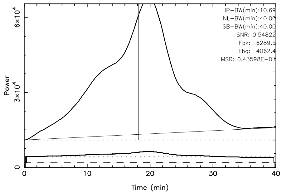
TOYOKAWA 3C392 2023/09/03(246)19:38:31-20:18:31JST
