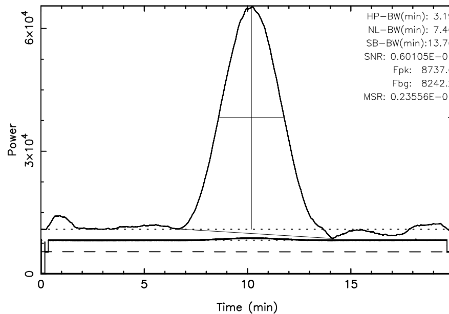
KISO 3C123 2023/10/03(276)03:34:11-03:54:10JST
