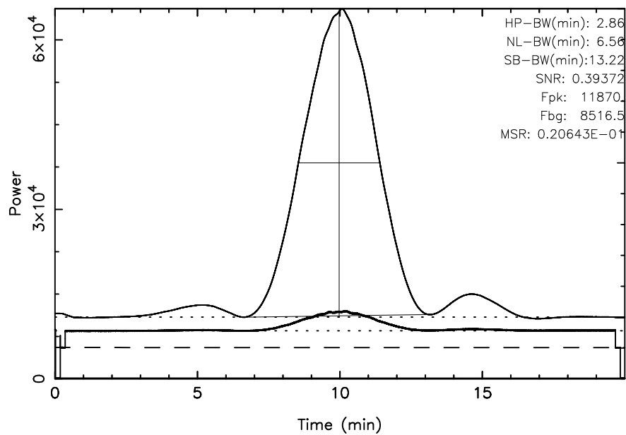
KISO 3C144 2023/10/03(276)04:31:23-04:51:23JST
