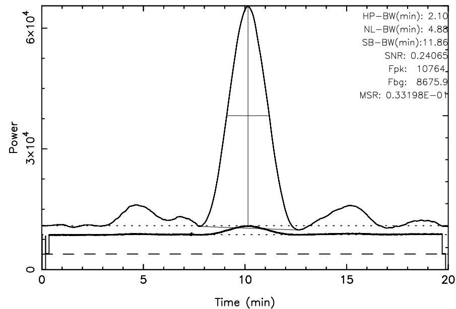
FUJI 3C144 2023/10/03(276)04:31:23-04:51:23JST
