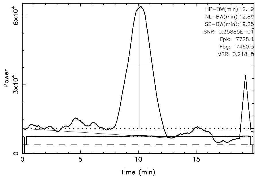
FUJI 3C123 2023/10/03(276)03:34:11-03:54:10JST
