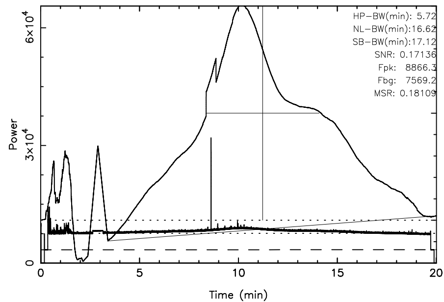
FUJI 3C392 2023/10/03(276)17:50:33-18:10:34JST
