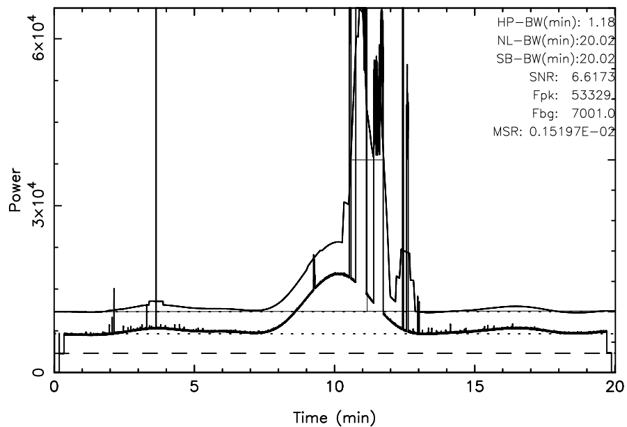
FUJI 3C405 2023/10/03(276)18:53:22-19:13:23JST
