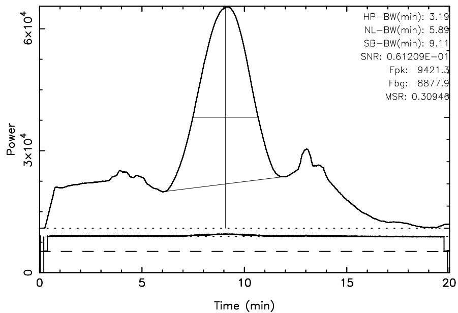
FUJI 3C157 2023/10/06(279)05:03:00-05:23:01JST
