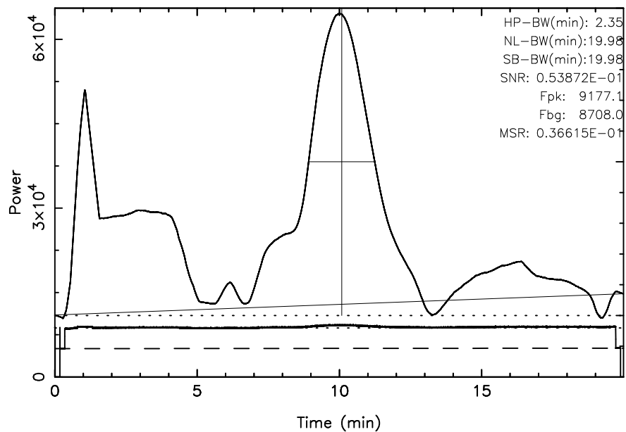
FUJI 3C123 2023/10/06(279)03:22:24-03:42:23JST
