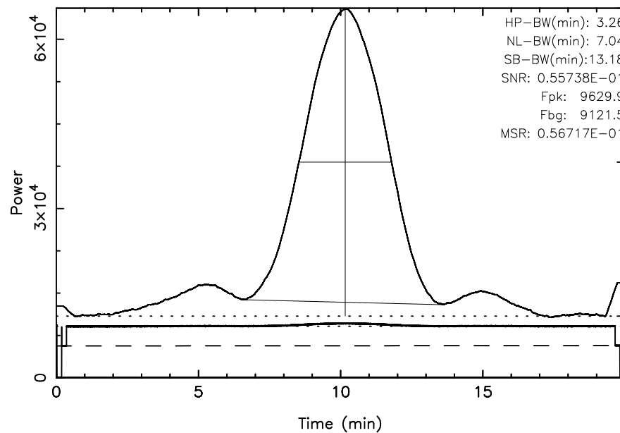
KISO 3C123 2023/10/06(279)03:22:24-03:42:23JST
