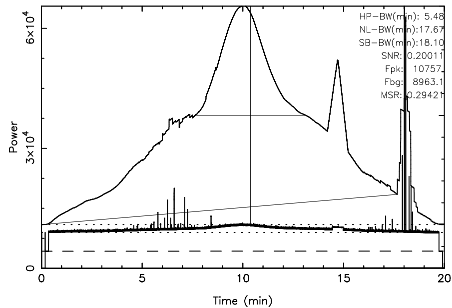
FUJI 3C392 2023/10/06(279)17:38:45-17:58:45JST
