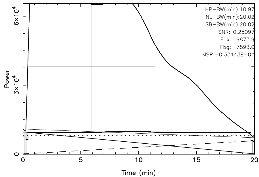
KISO 3C157 2023/10/06(279)05:03:00-05:23:01JST
