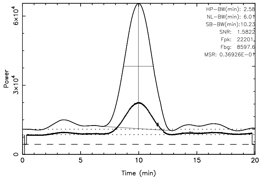
FUJI 3C405 2023/10/06(279)18:41:35-19:01:36JST
