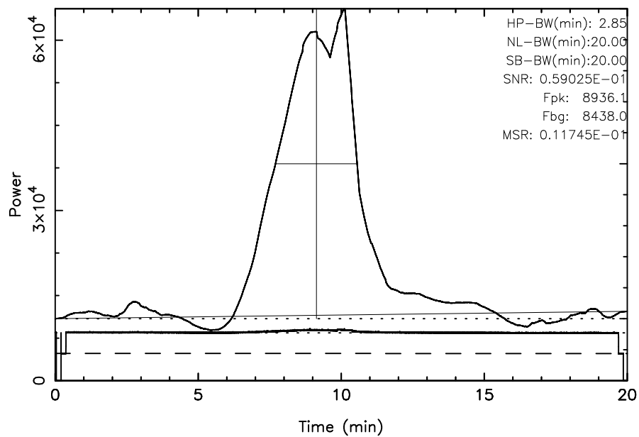
FUJI 3C157 2023/10/11(284)04:43:20-05:03:20JST
