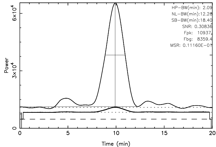
FUJI 3C144 2023/10/11(284)03:59:57-04:19:57JST
