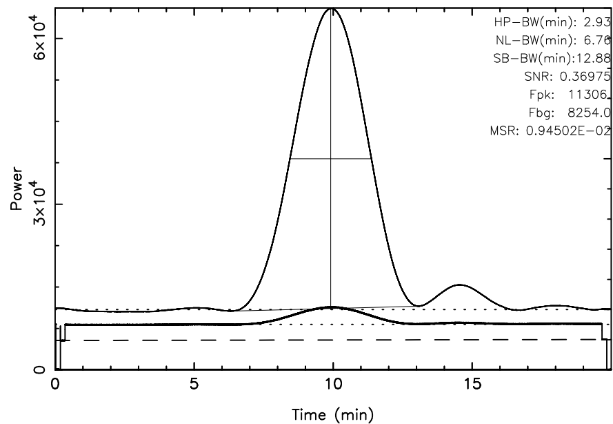
KISO 3C144 2023/10/11(284)03:59:57-04:19:57JST
