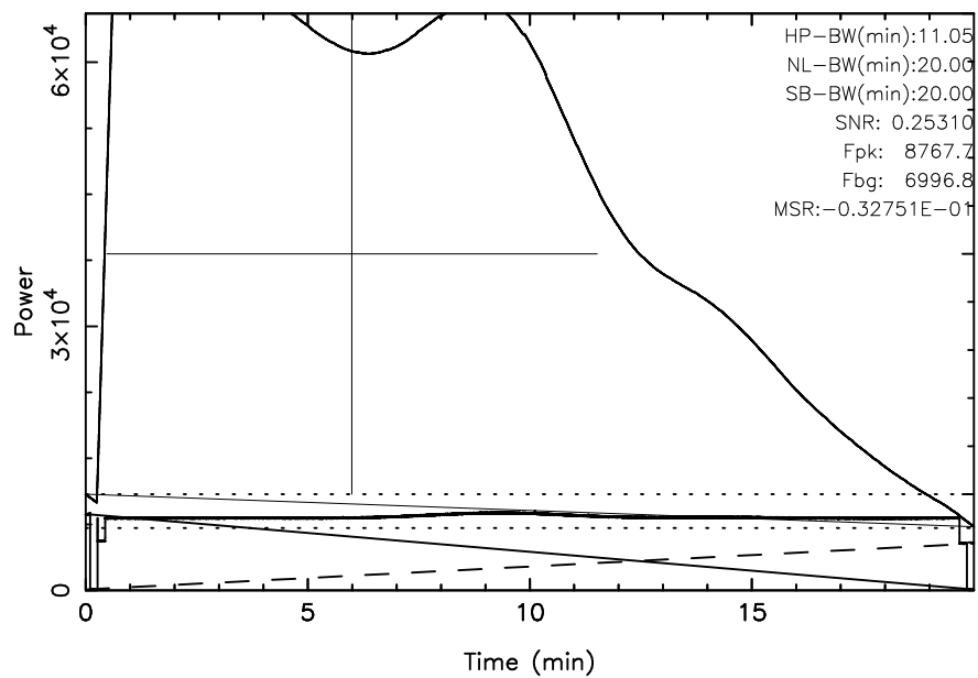
KISO 3C157 2023/10/11(284)04:43:20-05:03:20JST
