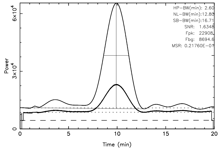
FUJI 3C405 2023/10/11(284)18:21:56-18:41:56JST
