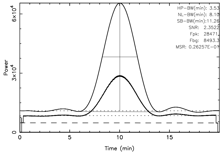
KISO 3C405 2023/10/11(284)18:21:56-18:41:56JST
