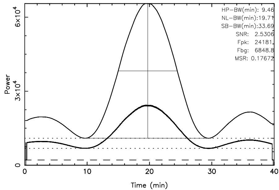
TOYOKAWA 3C461 2023/09/30(273)22:18:47-22:58:47JST
