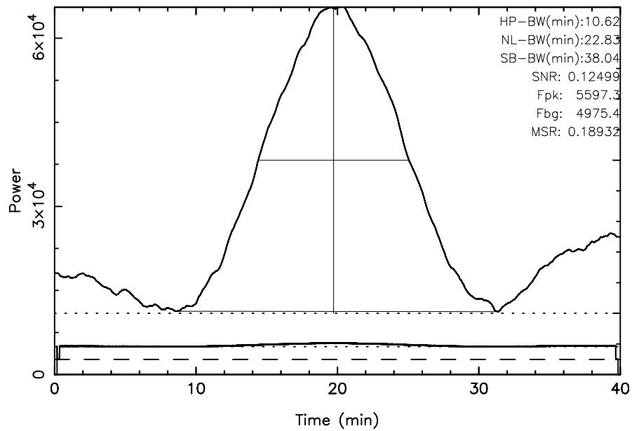
TOYOKAWA 3C10 2023/10/03(276)23:09:07-23:49:07JST
