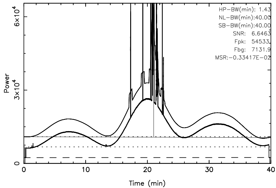
TOYOKAWA 3C405 2023/10/03(276)18:43:23-19:23:23JST
