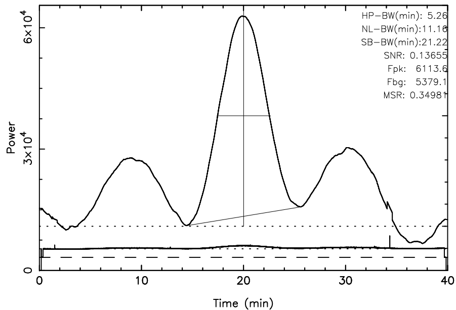
TOYOKAWA 3C123 2023/10/27(300)01:49:50-02:29:50JST
