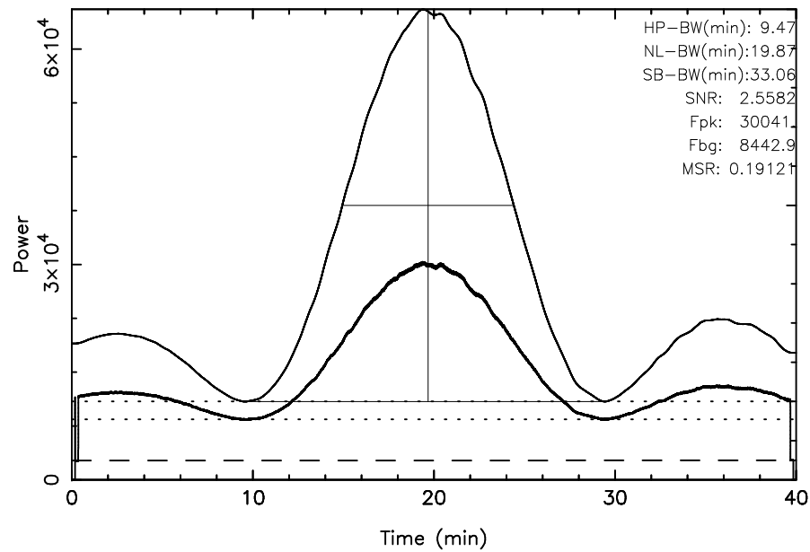
TOYOKAWA 3C461 2023/11/05(309)19:57:14-20:37:14JST
