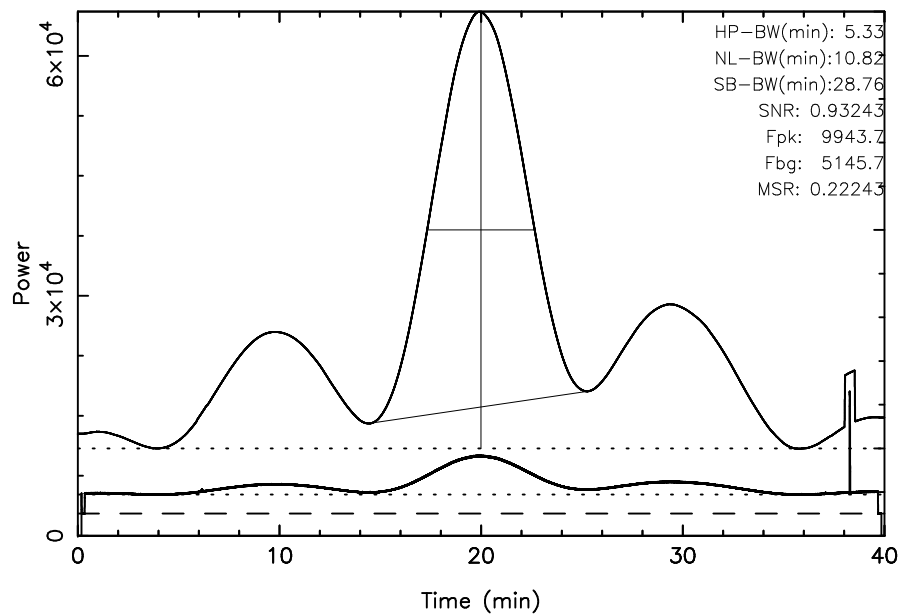
TOYOKAWA 3C144 2023/11/23(327)01:00:53-01:40:53JST
