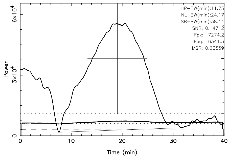
TOYOKAWA 3C10 2023/11/23(327)19:48:36-20:28:36JST
