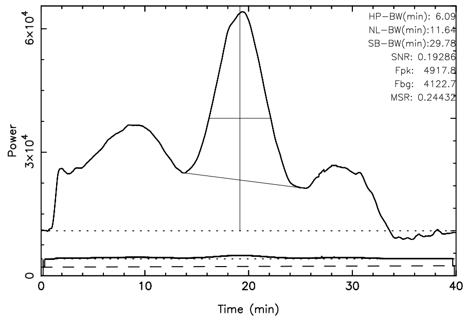
TOYOKAWA 3C157 2023/11/24(328)01:40:22-02:20:22JST
