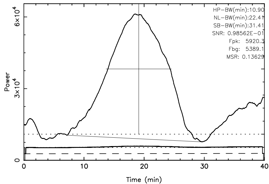
TOYOKAWA 3C10 2023/11/24(328)19:44:40-20:24:40JST
