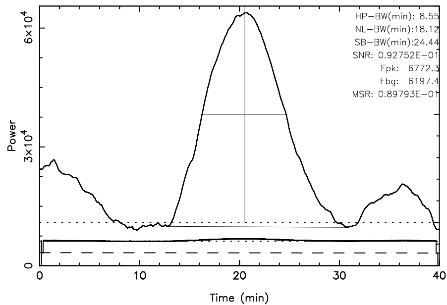
TOYOKAWA 3C10 2023/11/27(331)19:32:52-20:12:52JST
