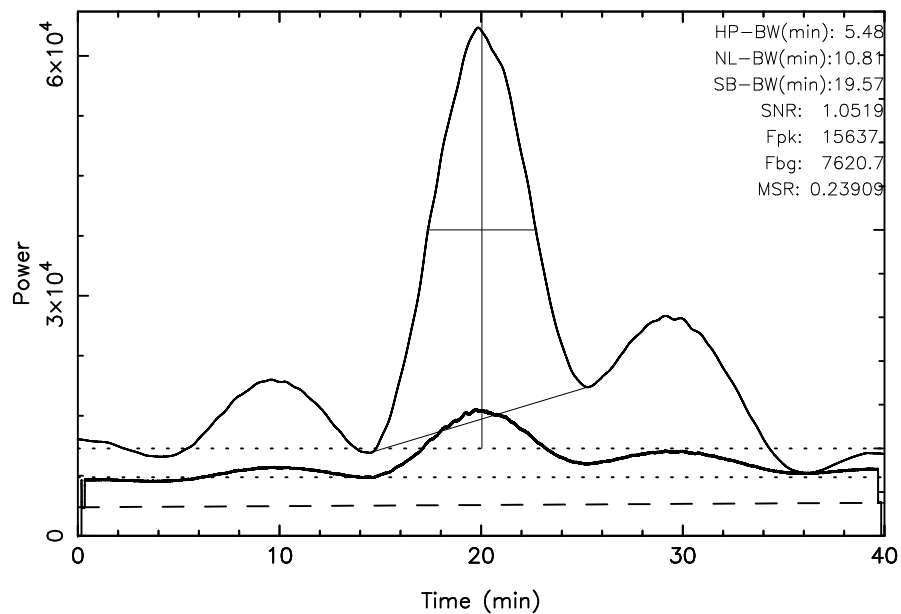
TOYOKAWA 3C144 2023/11/27(331)00:45:10-01:25:10JST
