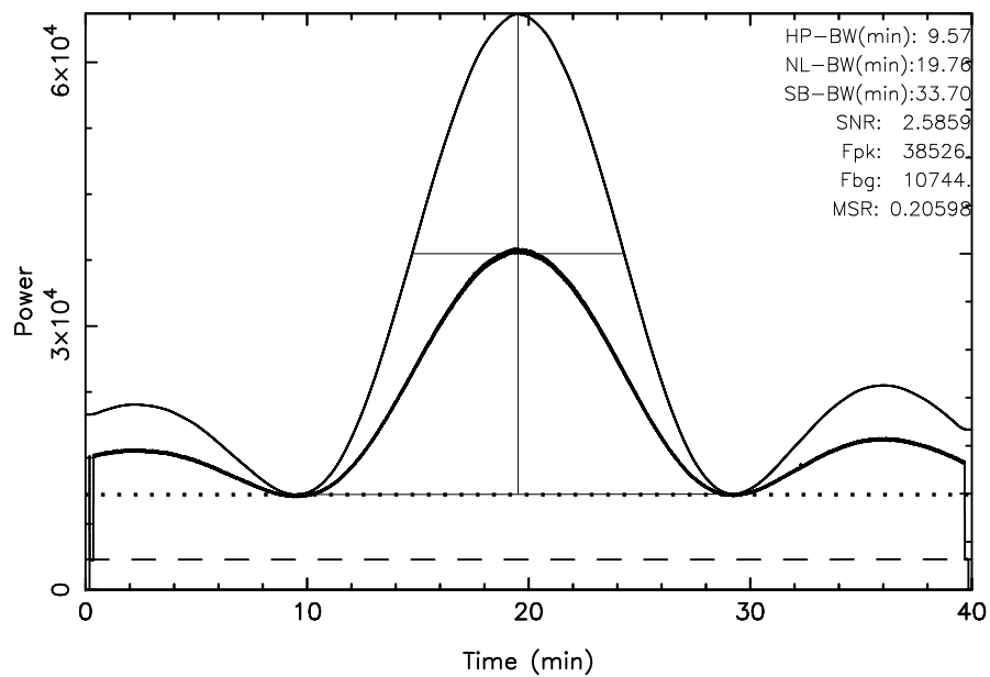
TOYOKAWA 3C461 2023/11/27(331)18:30:45-19:10:45JST
