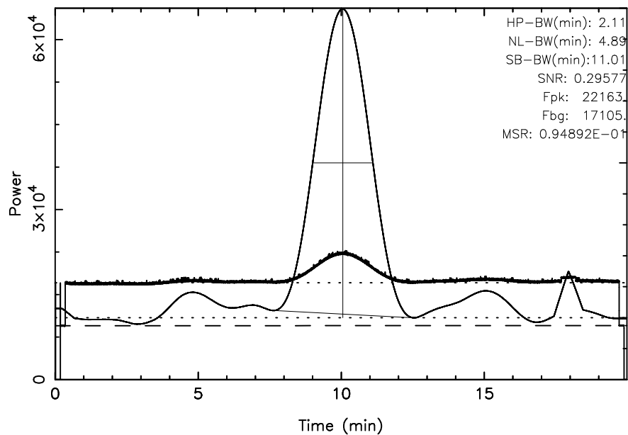
FUJI 3C144 2023/12/02(336)00:35:30-00:55:29JST
