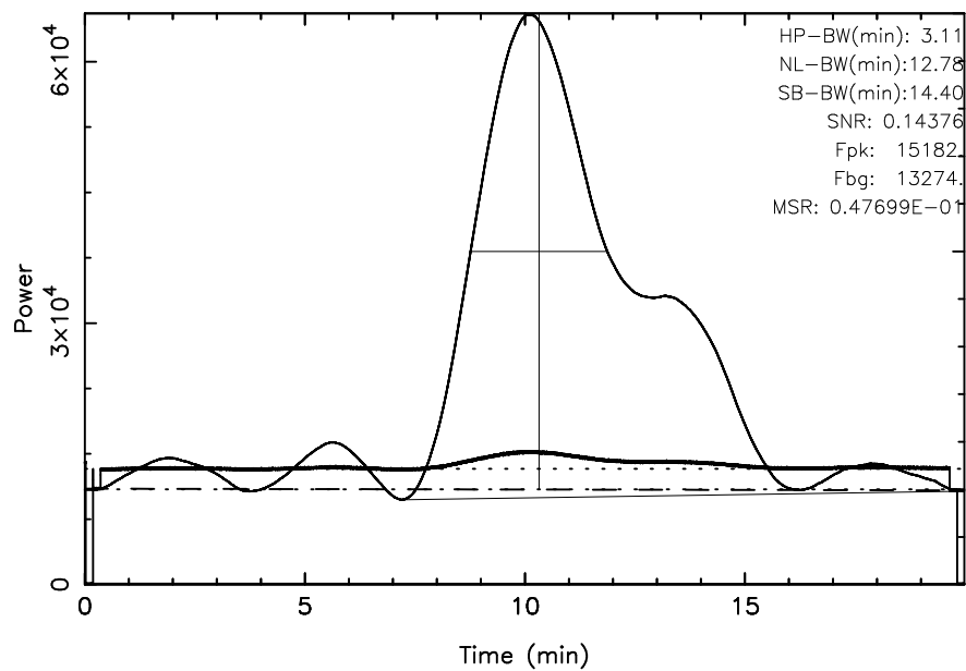
KISO 3C144 2023/12/02(336)00:35:30-00:55:29JST
