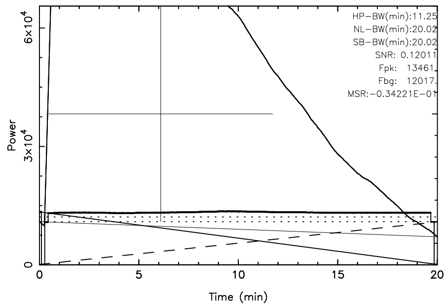
KISO 3C157 2023/12/02(336)01:18:53-01:38:54JST
