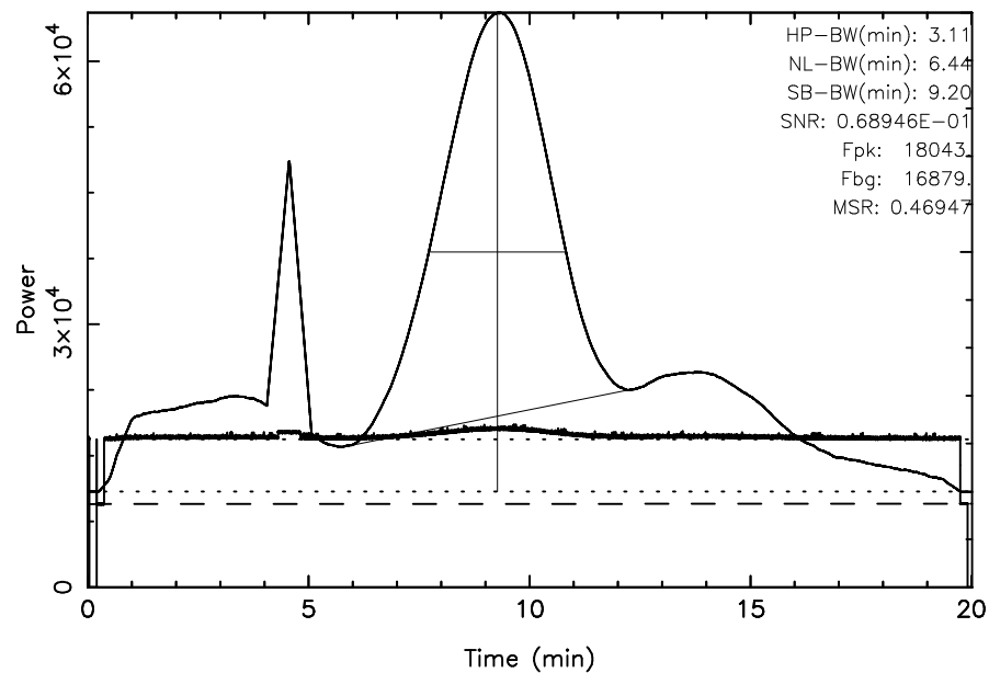
FUJI 3C157 2023/12/02(336)01:18:53-01:38:54JST
