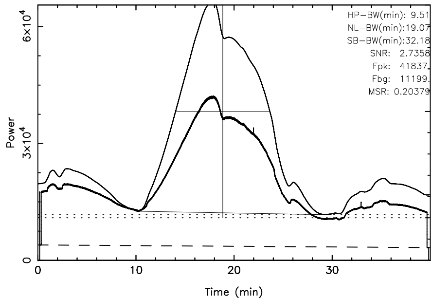
TOYOKAWA 3C461 2023/12/04(338)18:03:13-18:43:13JST
