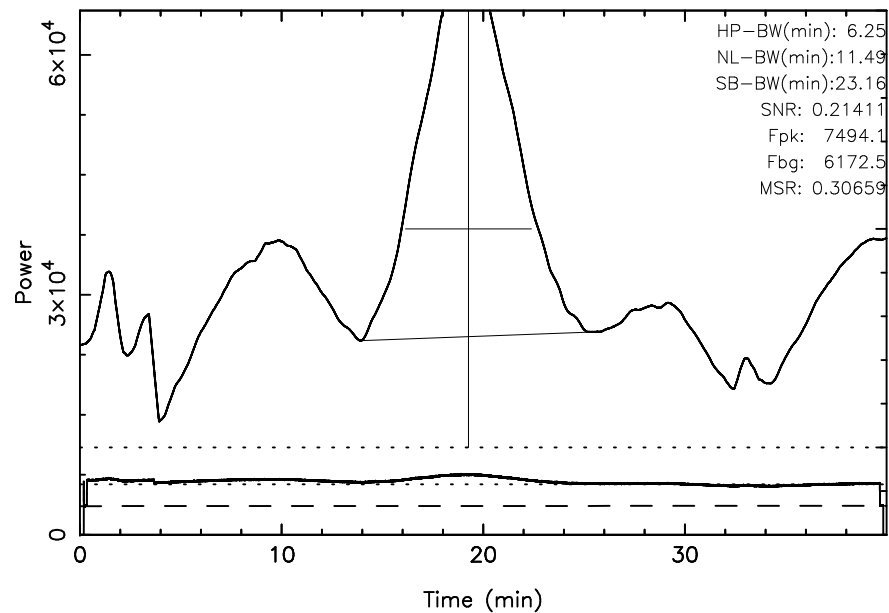
TOYOKAWA 3C157 2023/12/04(338)01:01:03-01:41:03JST
