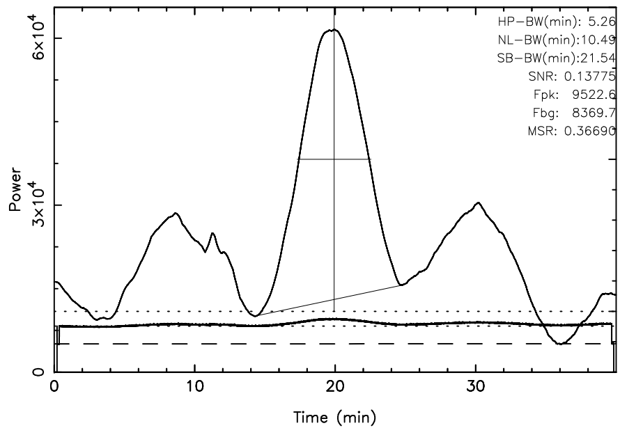
TOYOKAWA 3C123 2023/12/26(360)21:50:00-22:30:00JST
