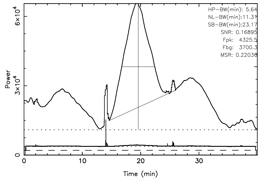
TOYOKAWA 3C157 2024/01/08(008)22:39:30-23:19:30JST
