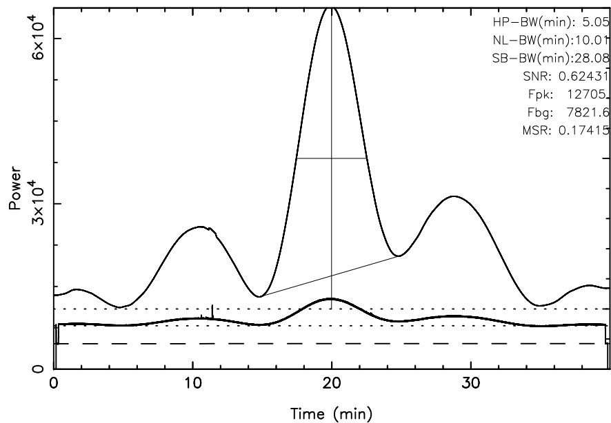
TOYOKAWA 3C274 2024/01/14(014)04:31:23-05:11:23JST
