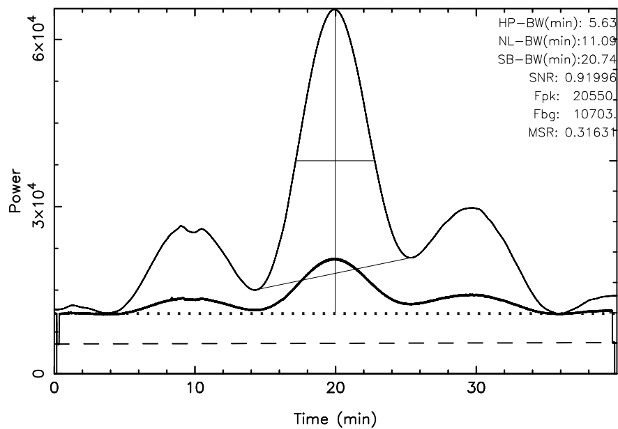
TOYOKAWA 3C144 2024/01/14(014)21:32:30-22:12:30JST
