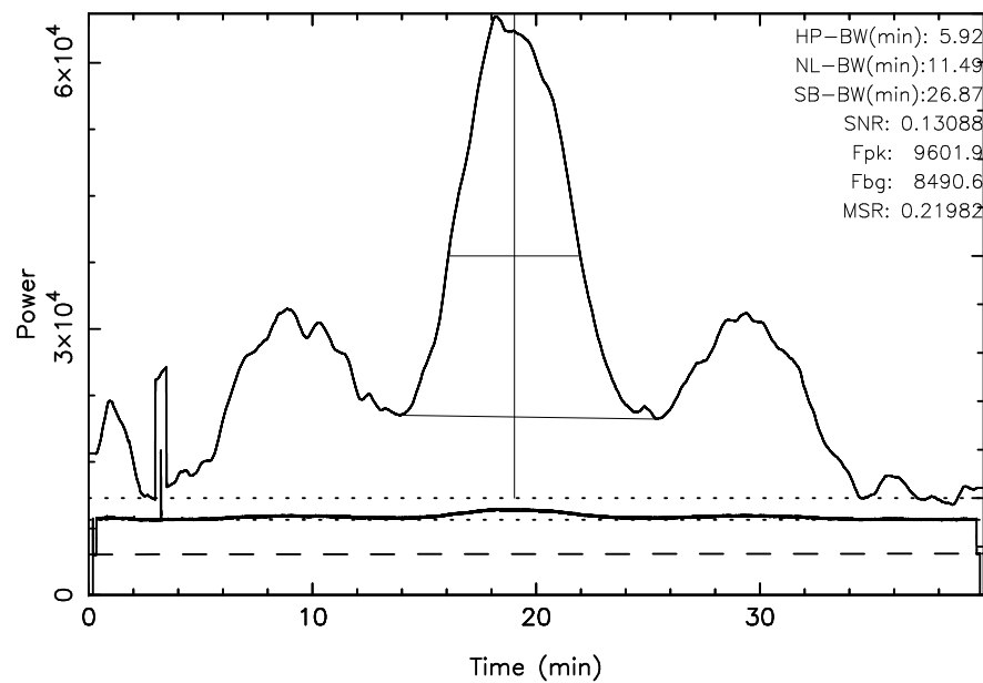
TOYOKAWA 3C157 2024/01/14(014)22:15:55-22:55:55JST
