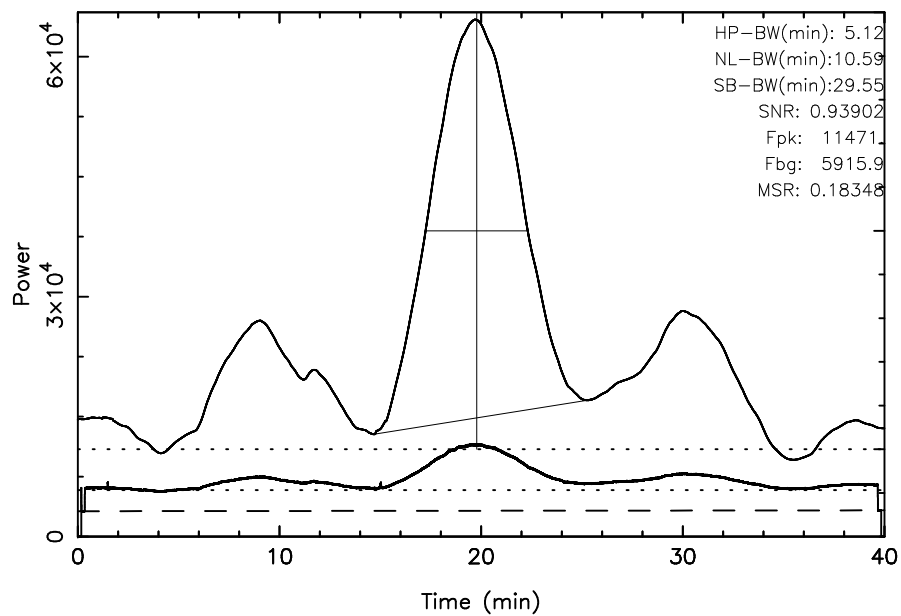
TOYOKAWA 3C144 2024/03/02(062)18:23:47-19:03:47JST
