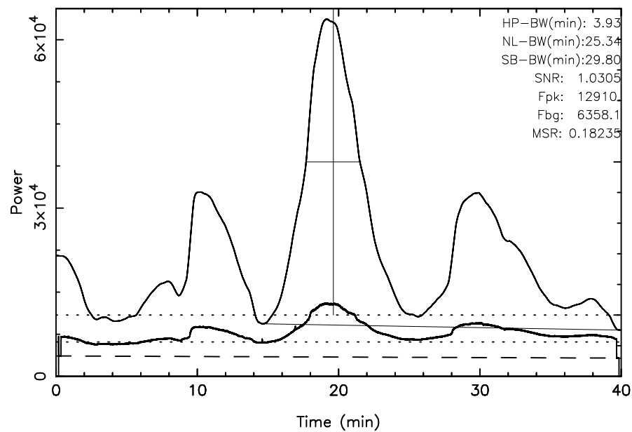
TOYOKAWA 3C144 2024/03/09(069)17:56:16-18:36:16JST
