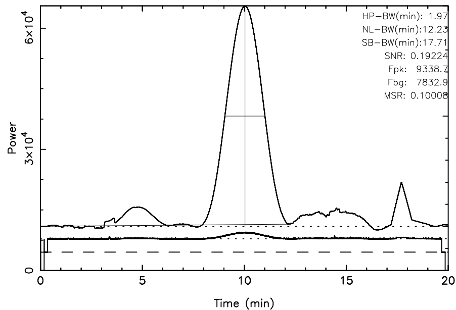
FUJI 3C274 2024/04/15(106)22:35:43-22:55:43JST
