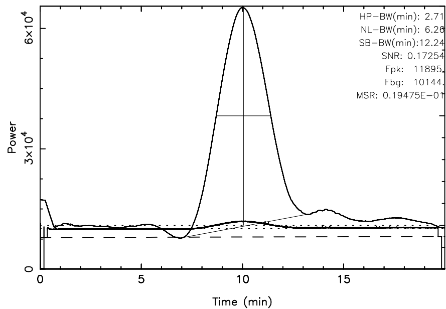
KISO 3C274 2024/04/15(106)22:35:43-22:55:43JST
