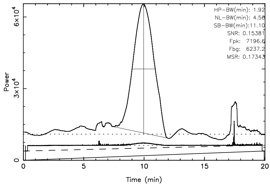
FUJI 3C274 2024/04/21(112)22:12:07-22:32:08JST
