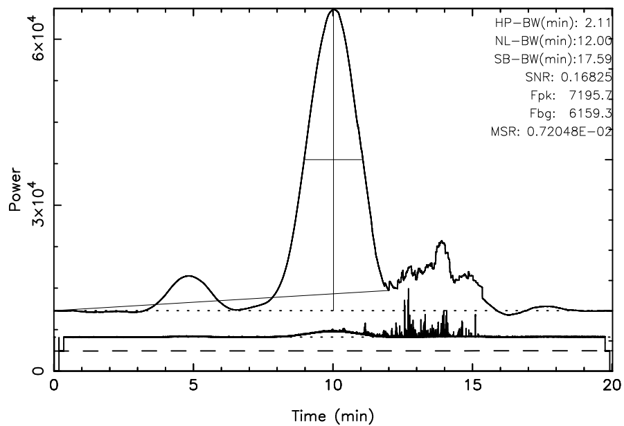
FUJI 3C274 2024/04/25(116)21:56:24-22:16:25JST
