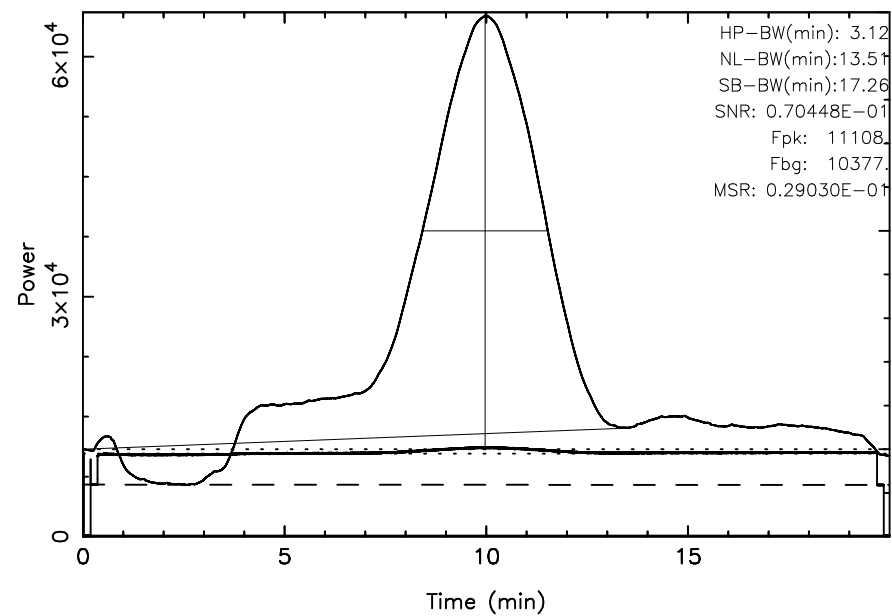
KISO 3C348 2024/04/25(116)02:19:55-02:39:55JST
