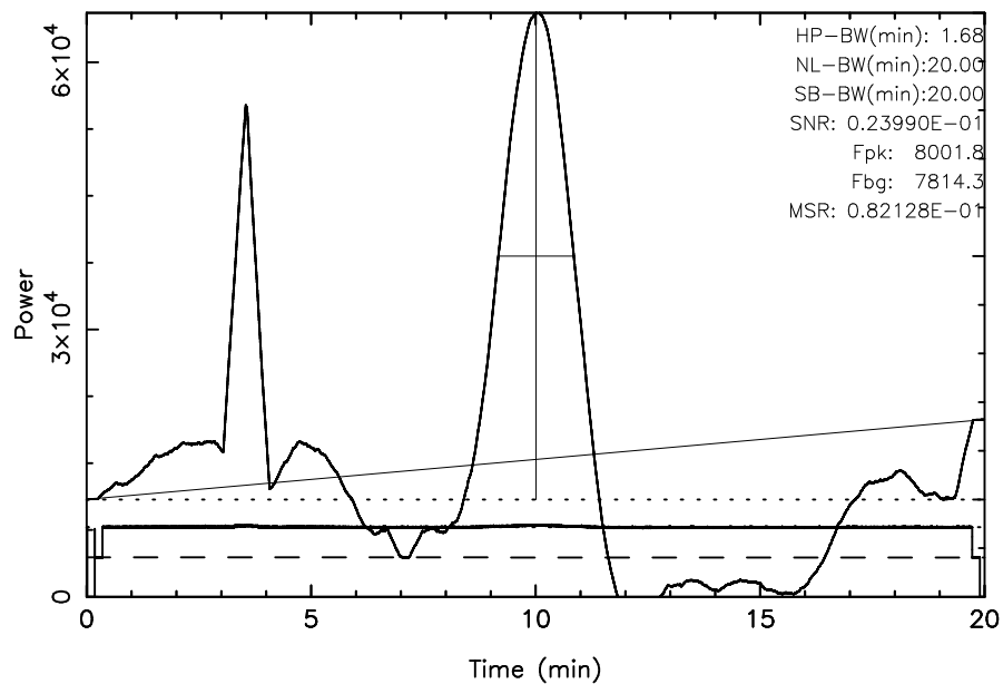
FUJI 3C348 2024/04/25(116)02:19:55-02:39:55JST
