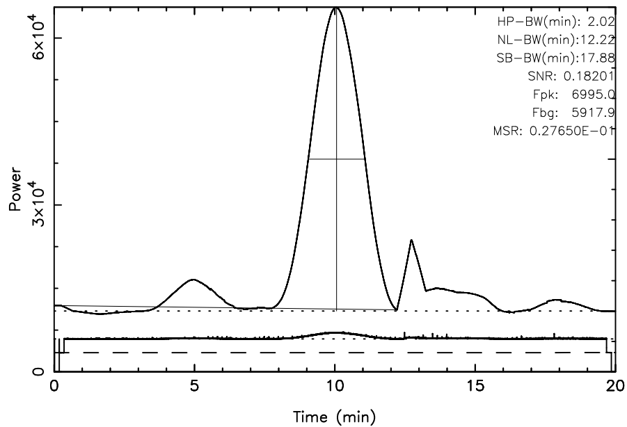
FUJI 3C274 2024/04/29(120)21:40:41-22:00:41JST
