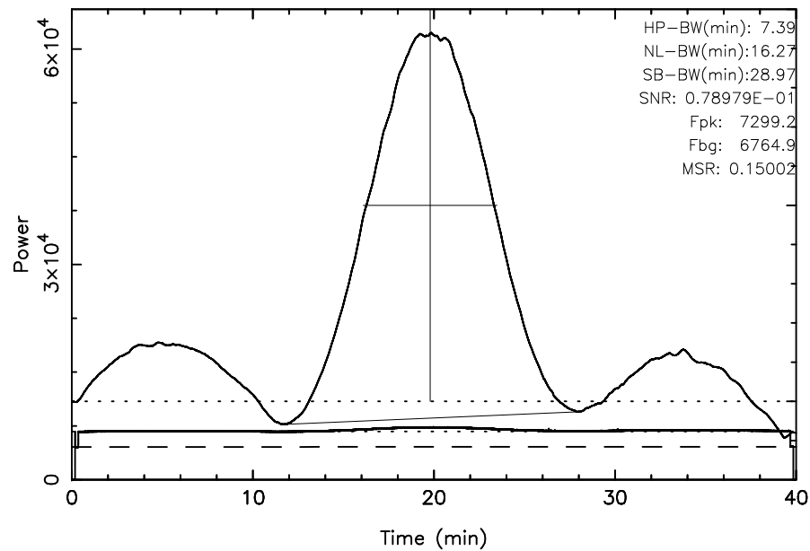
TOYOKAWA 3C295 2024/04/29(120)23:10:33-23:50:33JST
