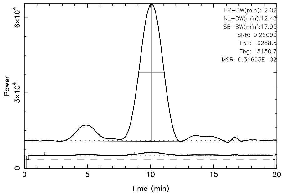
FUJI 3C274 2024/04/30(121)21:36:45-21:56:45JST
