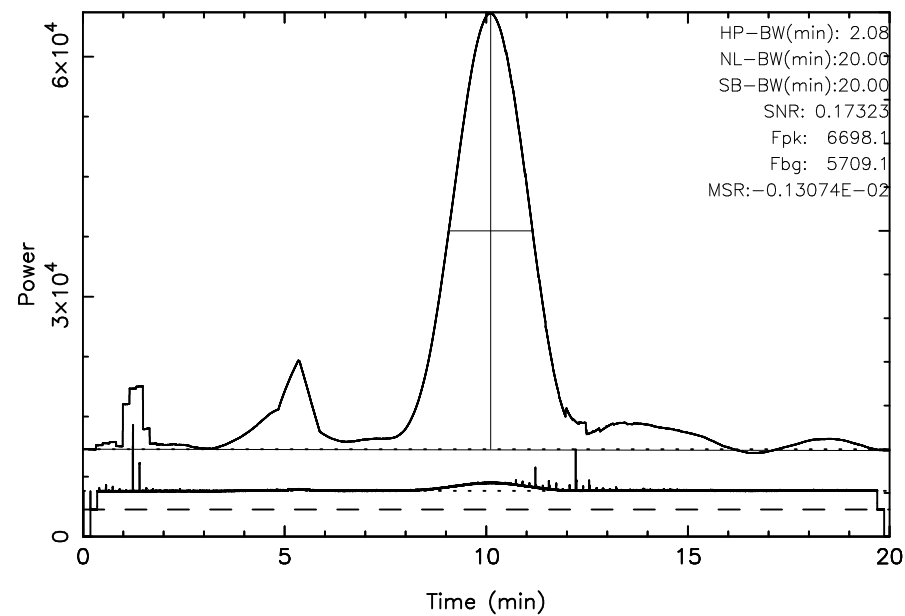
FUJI 3C274 2024/05/20(141)20:18:06-20:38:06JST
