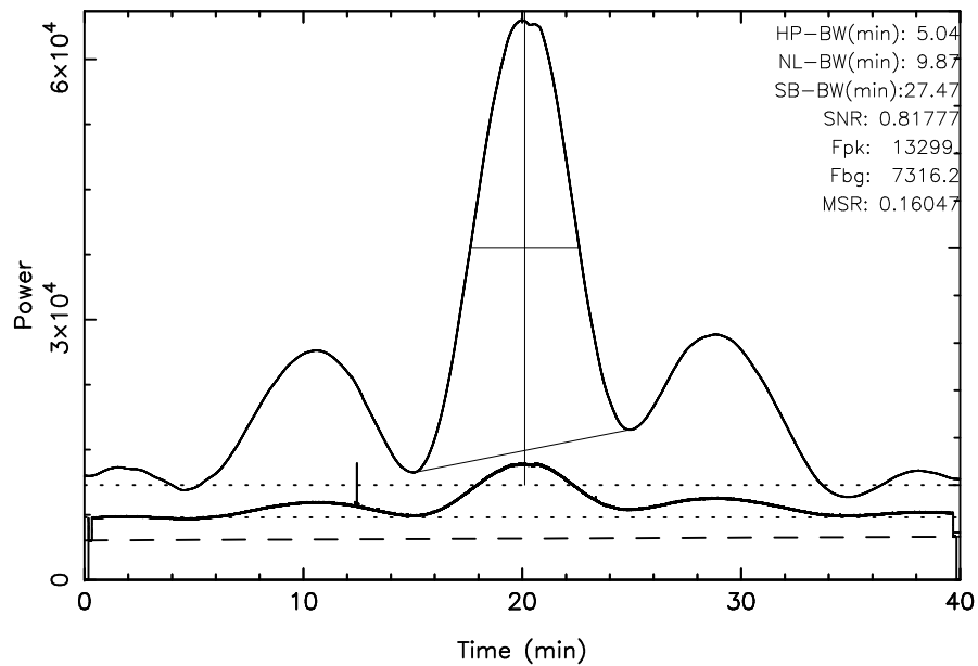
TOYOKAWA 3C274 2024/05/01(122)21:22:49-22:02:49JST
