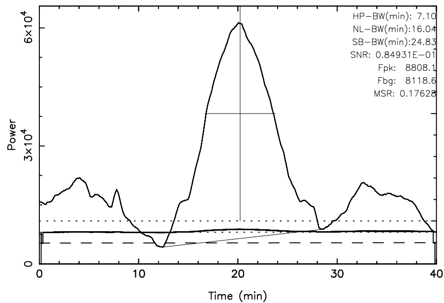
TOYOKAWA 3C295 2024/05/08(129)22:35:10-23:15:10JST
