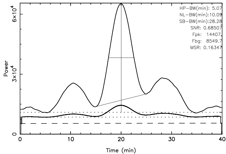
TOYOKAWA 3C274 2024/05/11(132)20:43:30-21:23:30JST
