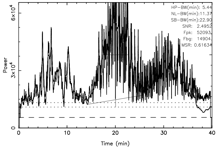
TOYOKAWA 3C405 2024/05/12(133)04:10:33-04:50:33JST
