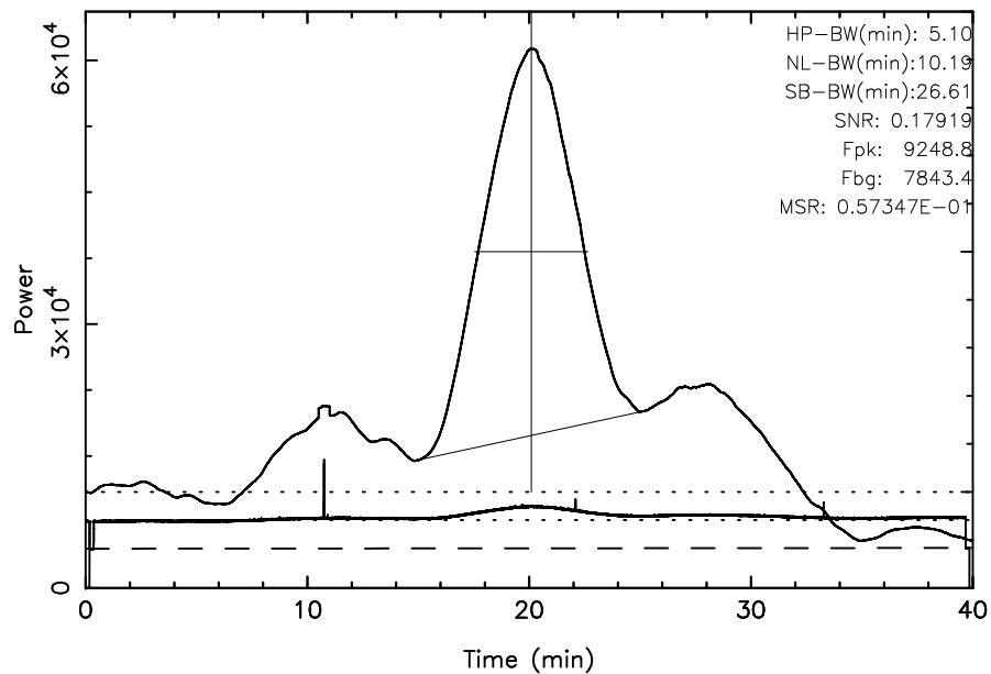
TOYOKAWA 3C348 2024/05/12(133)01:03:05-01:43:05JST
