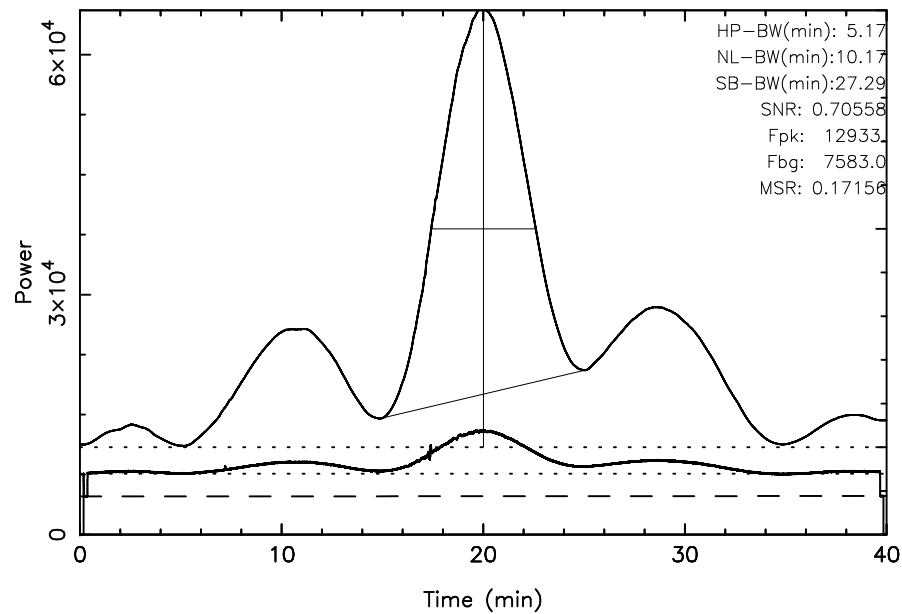
TOYOKAWA 3C274 2024/05/12(133)20:39:34-21:19:34JST
