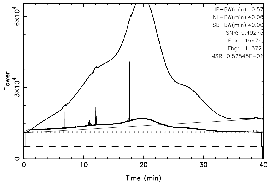
TOYOKAWA 3C392 2024/05/27(148)02:08:45-02:48:45JST
