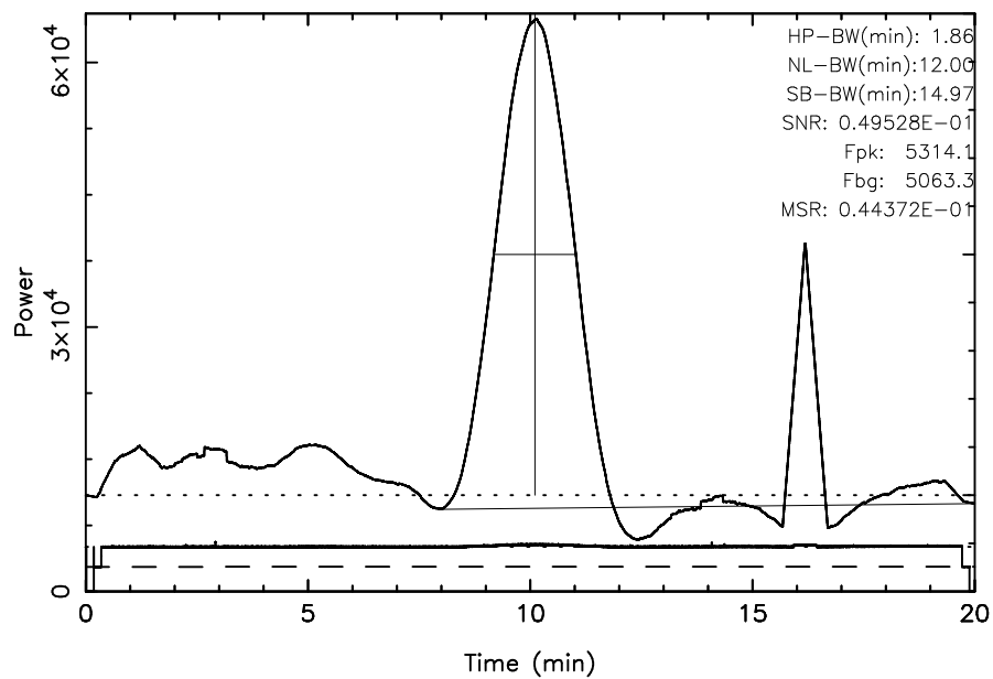
FUJI 3C348 2024/06/12(164)23:07:15-23:27:15JST
