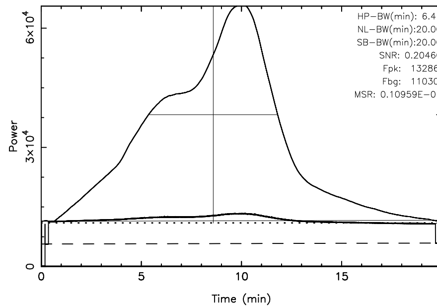
KISO 3C392 2024/06/12(164)01:15:50-01:35:50JST
