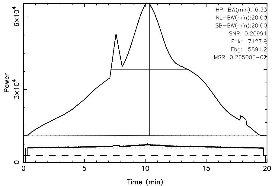
FUJI 3C392 2024/06/12(164)01:15:50-01:35:50JST
