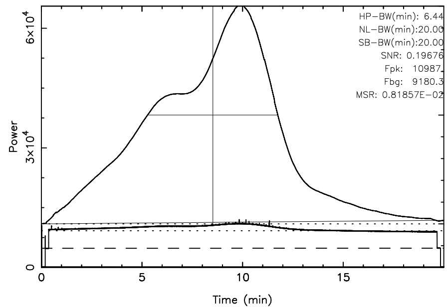
KISO 3C392 2024/07/20(202)22:42:30-23:02:30JST
