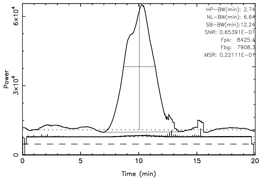
KISO 3C348 2024/07/20(202)20:37:51-20:57:52JST
