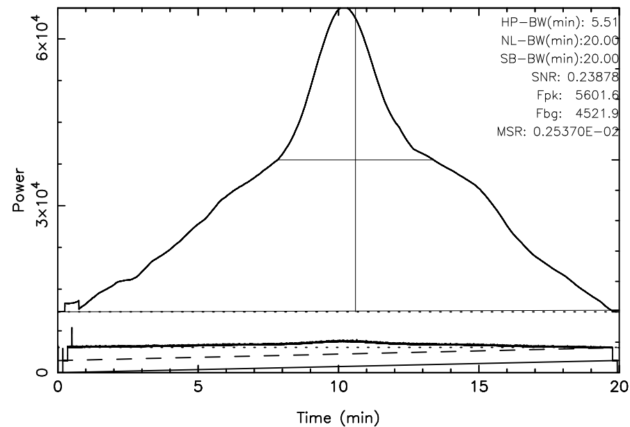
FUJI 3C392 2024/07/20(202)22:42:30-23:02:30JST
