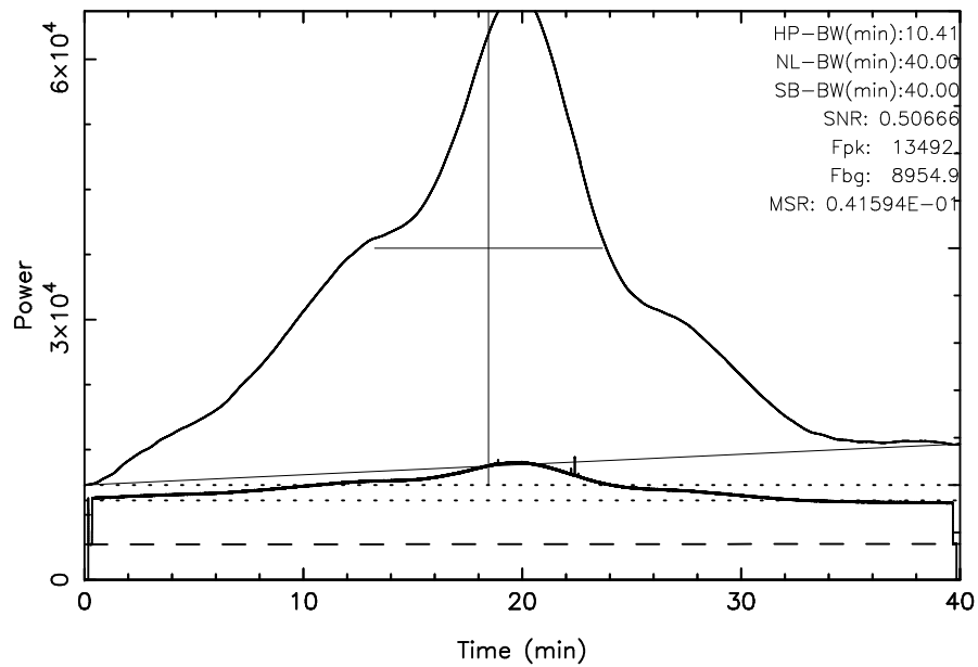
TOYOKAWA 3C392 2024/07/09(191)23:15:46-23:55:46JST
