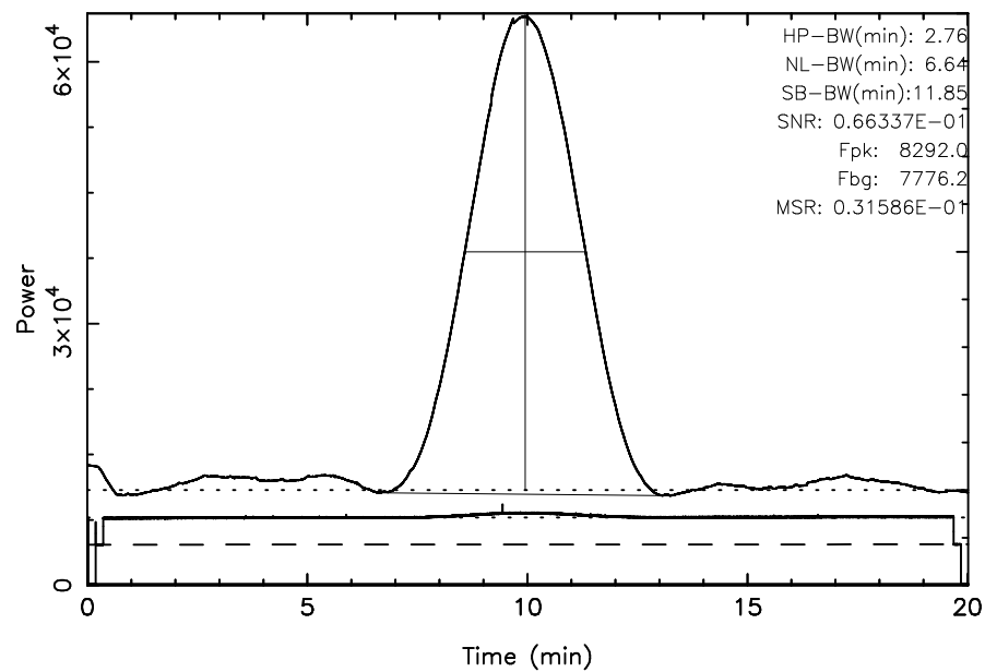
KISO 3C348 2024/08/02(215)19:46:44-20:06:45JST
