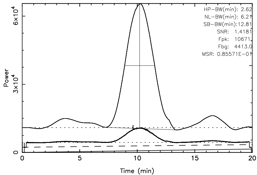
FUJI 3C405 2024/08/02(215)22:54:12-23:14:12JST
