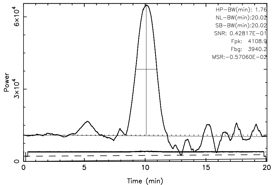
FUJI 3C348 2024/08/02(215)19:46:44-20:06:45JST
