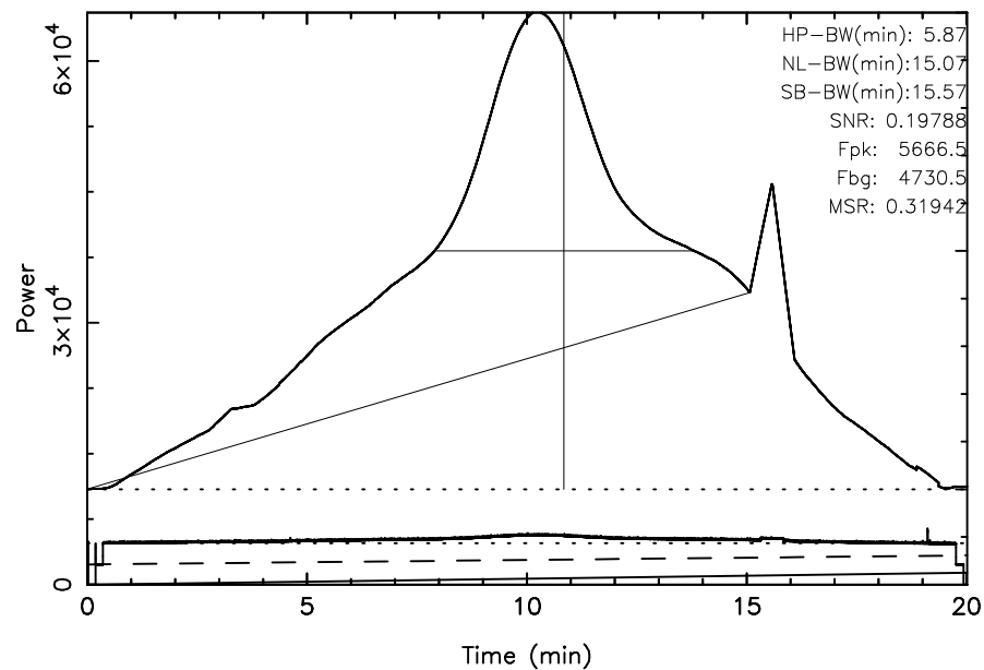
FUJI 3C392 2024/08/02(215)21:51:23-22:11:24JST
