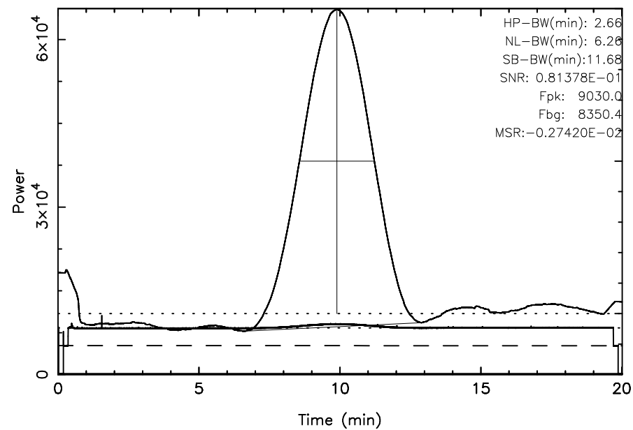
KISO 3C348 2024/08/08(221)19:23:09-19:43:10JST
