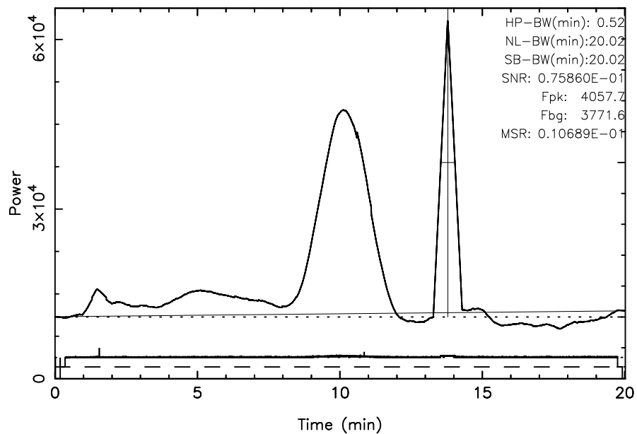
FUJI 3C348 2024/08/08(221)19:23:09-19:43:10JST
