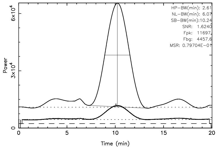
FUJI 3C405 2024/08/08(221)22:30:36-22:50:37JST
