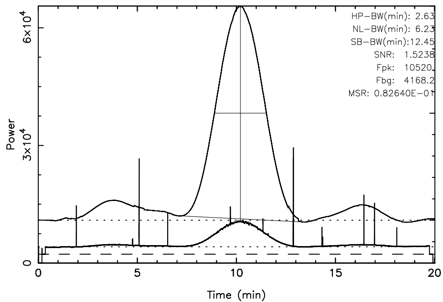
FUJI 3C405 2024/08/22(235)21:35:34-21:55:35JST
