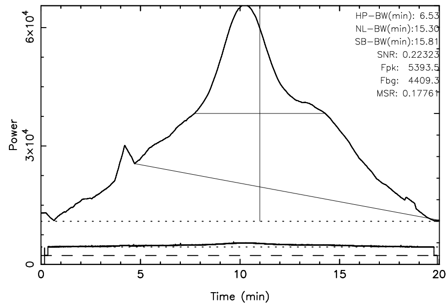
FUJI 3C392 2024/08/22(235)20:32:45-20:52:46JST
