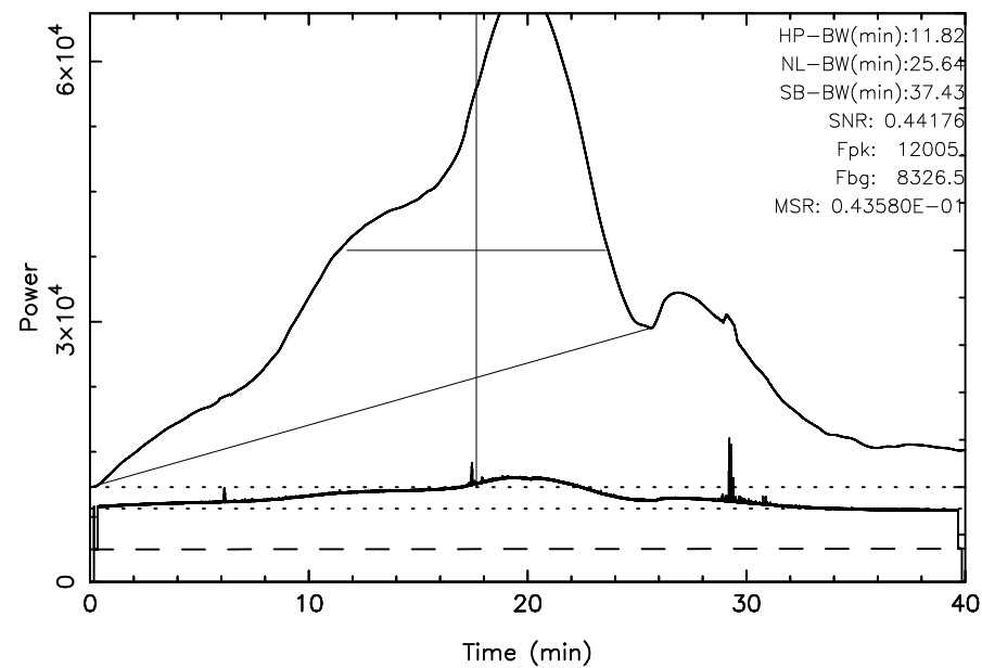
TOYOKAWA 3C392 2024/08/07(220)21:21:45-22:01:45JST
