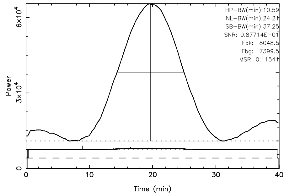
TOYOKAWA 3C10 2024/08/07(220)02:54:14-03:34:14JST
