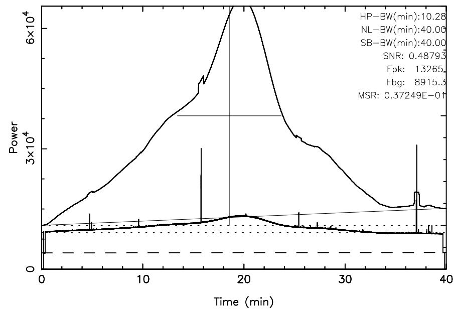
TOYOKAWA 3C392 2024/08/12(225)21:02:05-21:42:05JST
