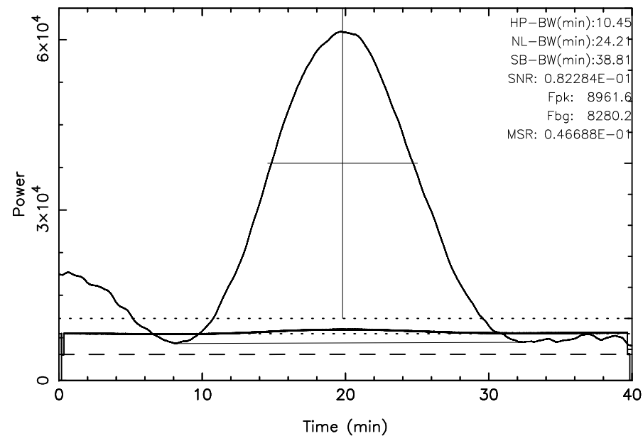
TOYOKAWA 3C10 2024/08/12(225)02:34:34-03:14:34JST
