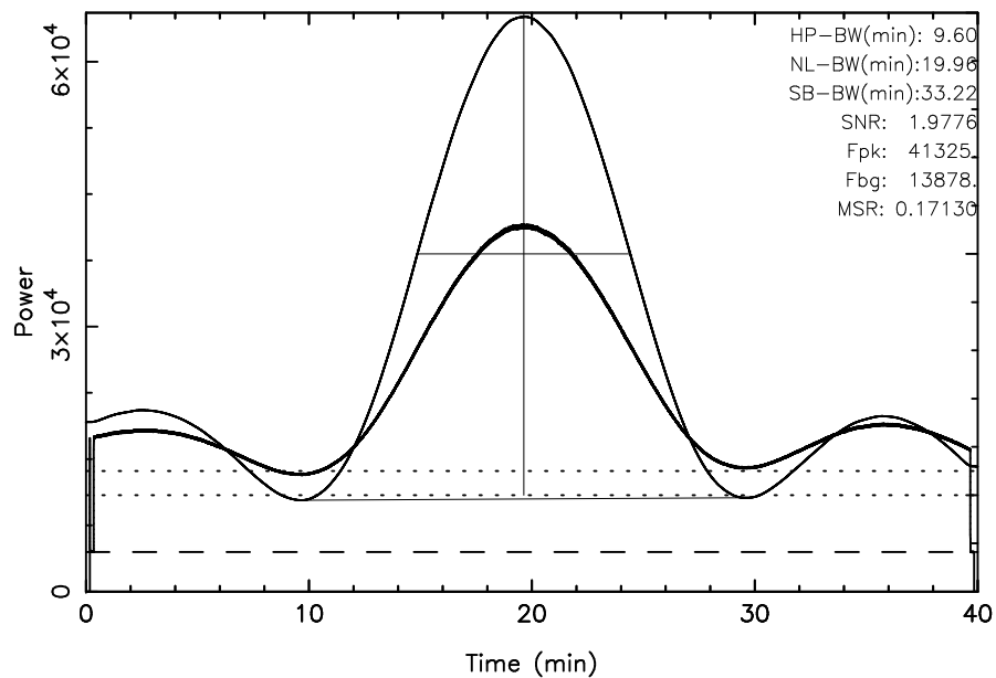
TOYOKAWA 3C461 2024/08/12(225)01:32:26-02:12:26JST
