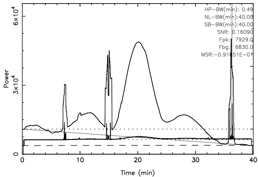
TOYOKAWA 3C348 2024/08/12(225)18:57:26-19:37:26JST
