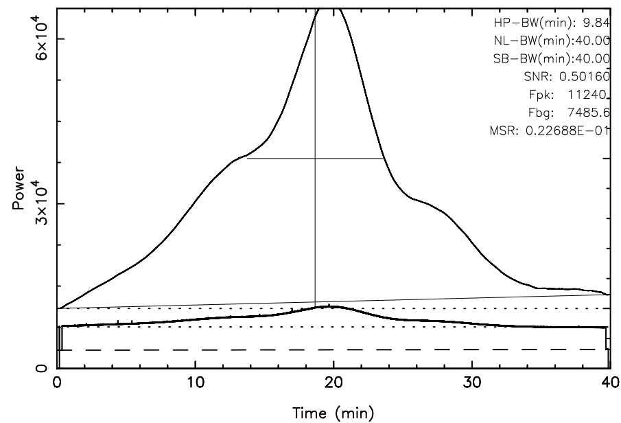
TOYOKAWA 3C392 2024/08/22(235)20:22:46-21:02:46JST
